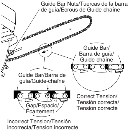
Figure 7 - Saw Chain Adjustment Figura 7 - Ajuste de la cadena serrada Figure 7 - Réglage de la chaîne
